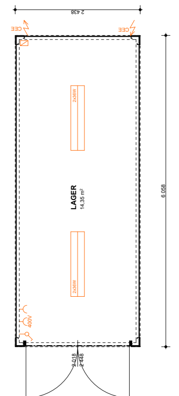
SK2 Flatpack - mit Elektro
