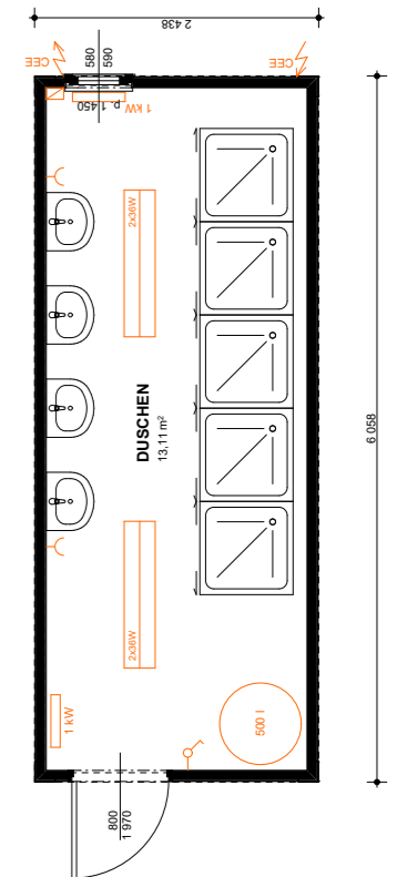
SK2 Flatpack - mit Elektro
