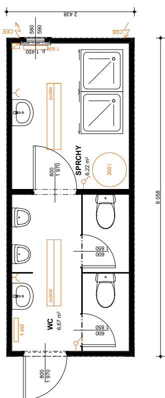
SA3 Sanitární modul - kombinovaný
