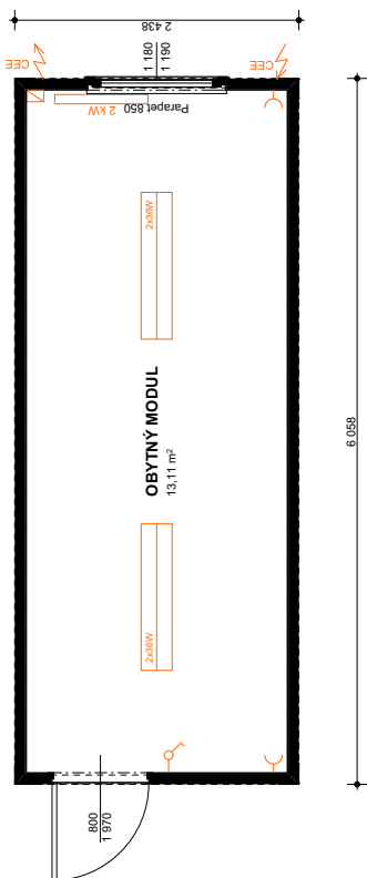
OB1 Obytný modul
