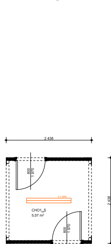
CHO1 Chodbový modul
