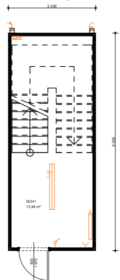
SCH1 Schodišťový modul
