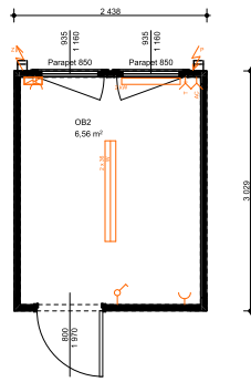
SA3 Kombinovaný modul
