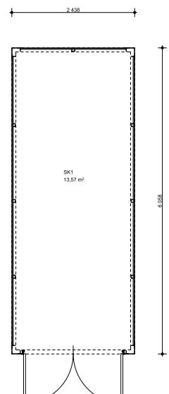
SK1 Skladový modul bez elektra
